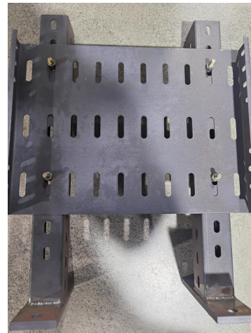
耐火试验-测试后
