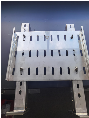
耐火试验-测试前
